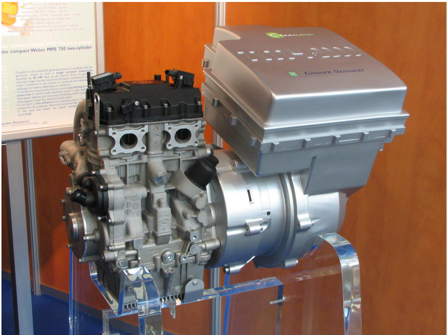
Kombinierter seriell und parallel Hybridmotor vom Renault Kangoo Cleanova II gezeigt auf der EVER Monaco 2007.
