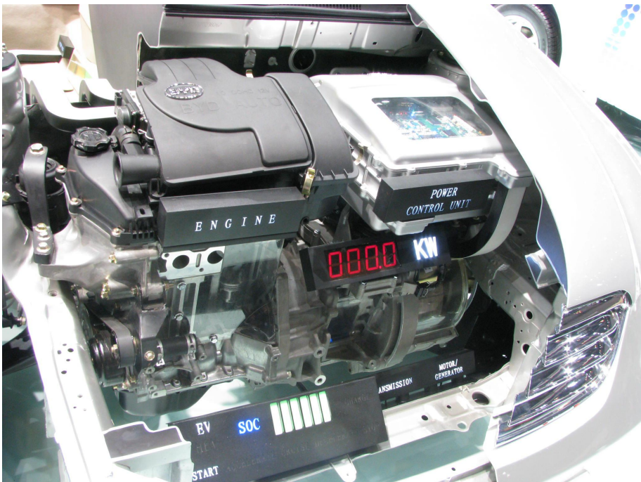
BYD F3DM seriell parallel hybrid System: Links der Verbrennungsmotor, rechts der Motorkontroller, darunter der Elektromotor.
